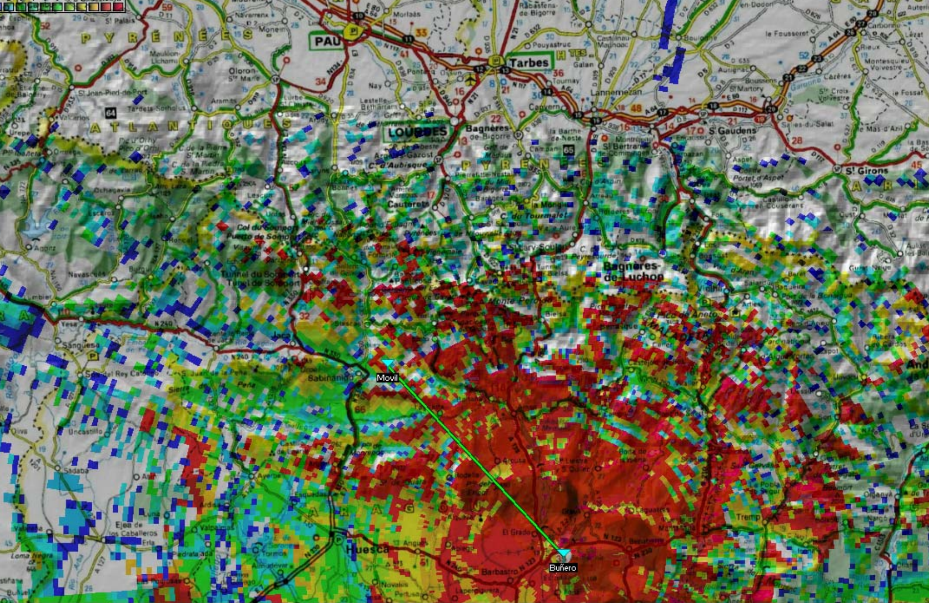
COBERTURA TEÓRICA R-4 BUÑERO (REMER HUESCA)
